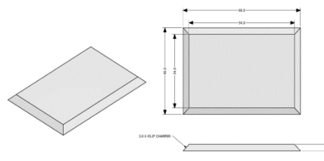
Gambar 2. Alas Kerangka
