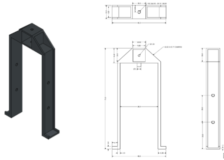
Gambar 3. Kerangka Penopang Sumber: (Penulis, 2025)
