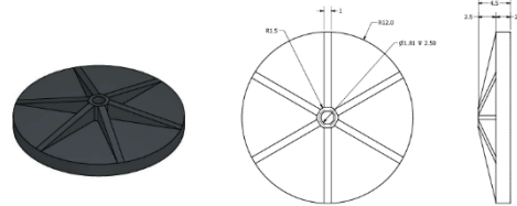
Gambar 7. Saringan Pres Sumber: (Penulis, 2025)
