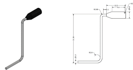
Gambar 8. Tuas Pengungkit Sumber: (Penulis, 2025)
